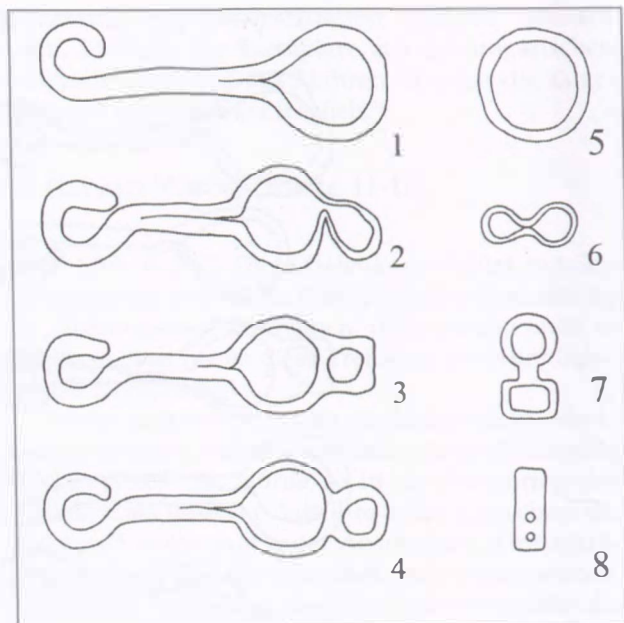
Abb. 47 Umgestaltung der Mundseitenringe und anschließenden Zaum/Zügelglieder und ihre Varianten:
