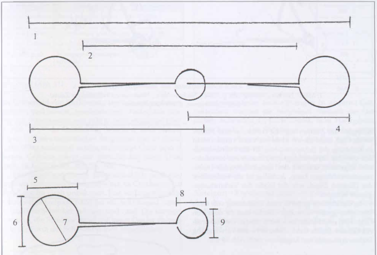
Abb. 48 Trensenmaße: A-Mundeisen – beide Endringe in identischer Ebene; B-Mundeisen – Ebene des inneren Scharnierreinges weicht 90° von der des äußeren Endringes ab; 1: größte Länge; 2: innere sog. physiologische L; 3: L des A-Mundeisens (Trensengliedes); 4: L des B-Mundeisens (Trensengliedes); 5: L des äußeren Endringes; 6: B des äußeren Endringes; 7: Innen-Dm. des äußeren Endringes; 8: L des inneren Endringes; 9: B des inneren Endringes
